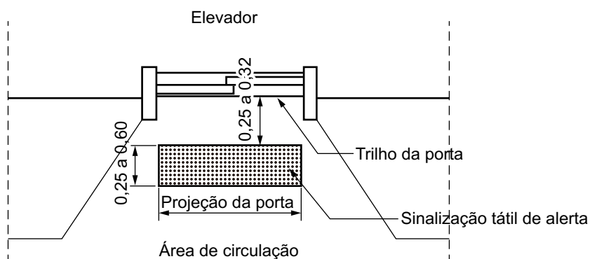
Figura 41 – Elevador com alvenaria chanfrada
