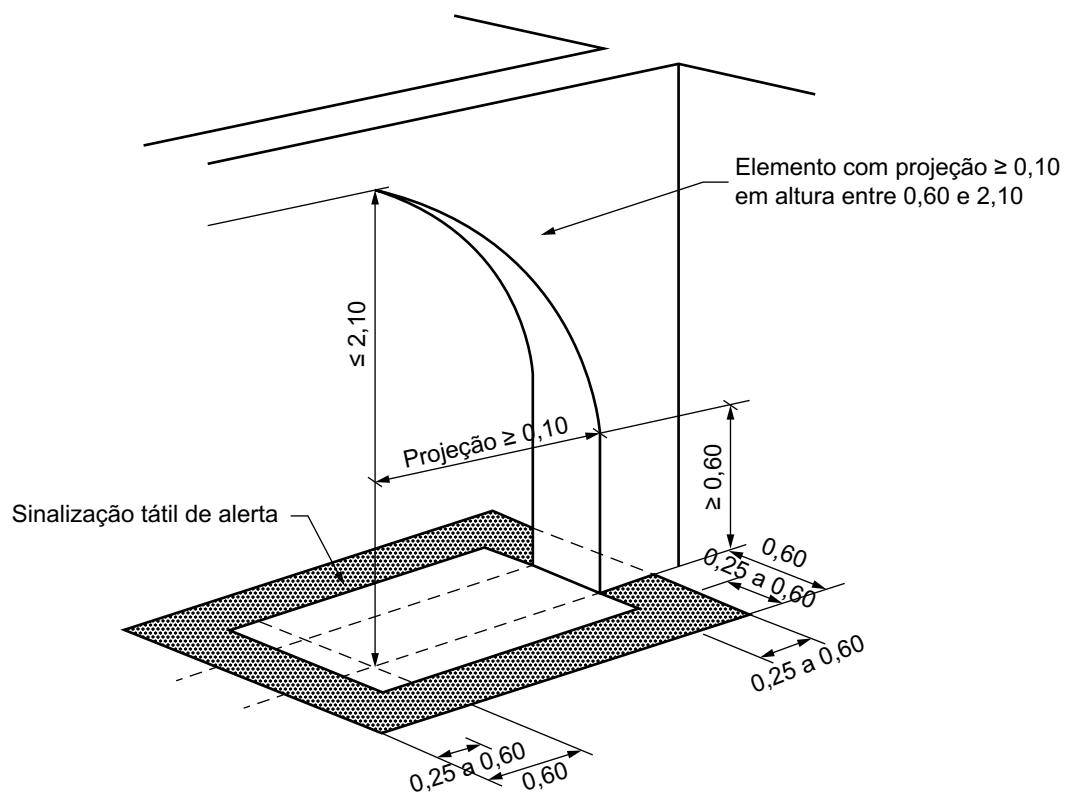
Figura 36 – Elemento construtivo
