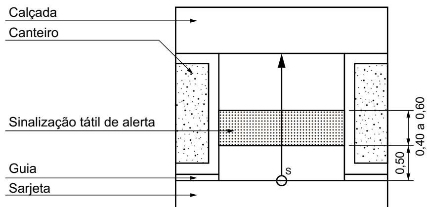
Figura 25 – Rebaixamento de calçada com canteiro
